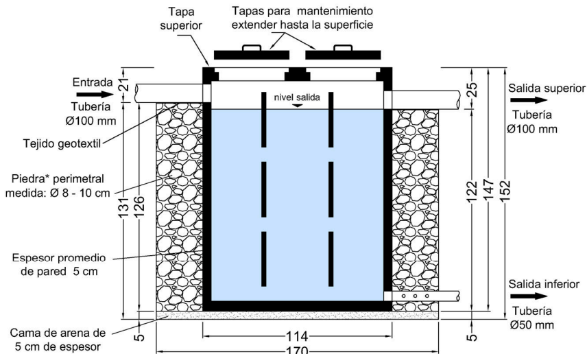
Tanque de Retardo Pluvial T.D. Modelo TRP-950 con piedra perimetral sección vertical - medidas en cm ©TANQUE DIEZ - Derechos Reservados
