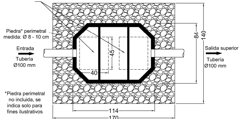
Tanque de Retardo Pluvial T.D. Modelo TRP-950 con piedra perimetral sección horizontal - medidas en cm ©TANQUE DIEZ - Derechos Reservados
