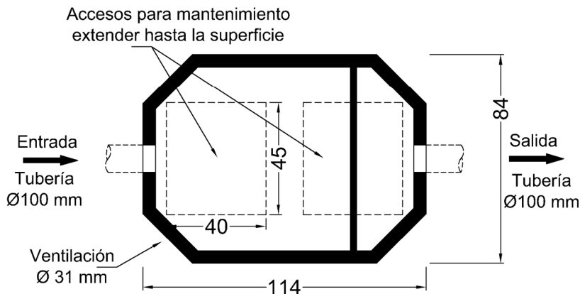
Sedimentador / Desarenador T.D. Modelo SPD-500 sección horizontal - medidas en cm
