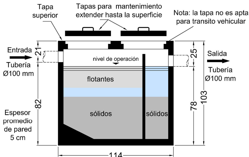
Sedimentador / Desarenador T.D. Modelo SPD-500 sección vertical - medidas en cm
