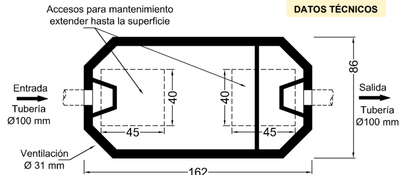
Sedimentador / Desarenador T.D.
