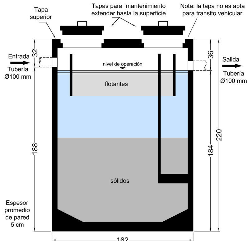
Sedimentador / Desarenador T.D.
