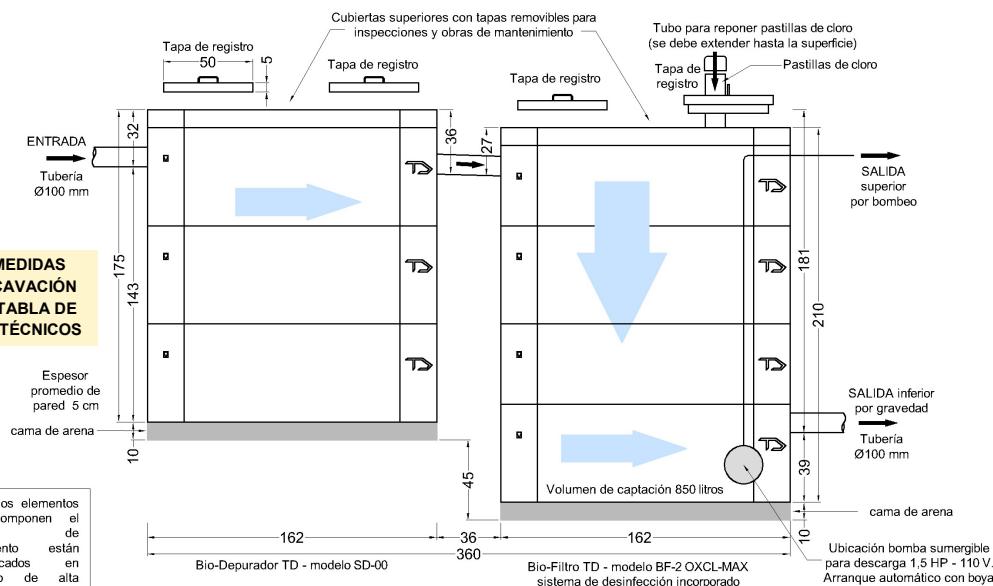
SISTEMA DE TRATAMIENTO TANQUE DIEZ MODELO PTB-OX15 - CAUDAL DIARIO A TRATAR 1,5 M 3 VISTA VERTICAL DE LAS UNIDADES DE TRATAMIENTO - MEDIDAS EN CENTÍMETROS TANQUE DIEZ - DERECHOS RESERVADOS
