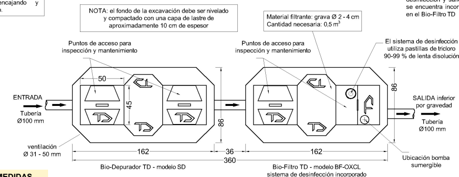
SISTEMA DE TRATAMIENTO TANQUE DIEZ MODELO PTB-OX15 - CAUDAL DIARIO A TRATAR 1,5 M 3 VISTA SUPERIOR DE LAS UNIDADES DE TRATAMIENTO - MEDIDAS EN CENTÍMETROS TANQUE DIEZ - DERECHOS RESERVADOS
