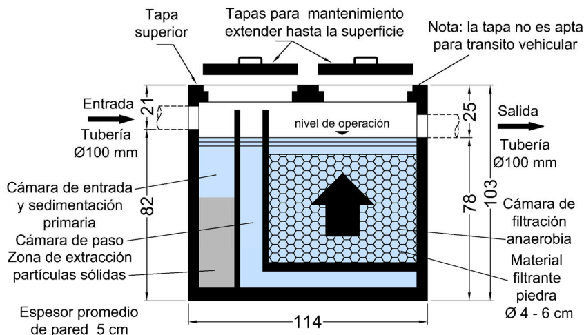
Filtro Anaerobio de Flujo Ascendente T.D.
