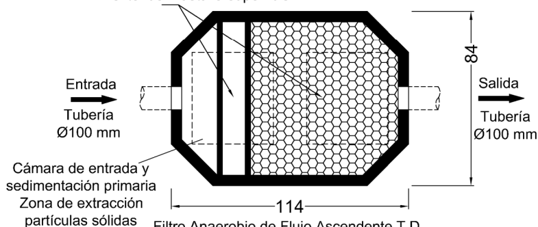
Filtro Anaerobio de Flujo Ascendente T.D.
