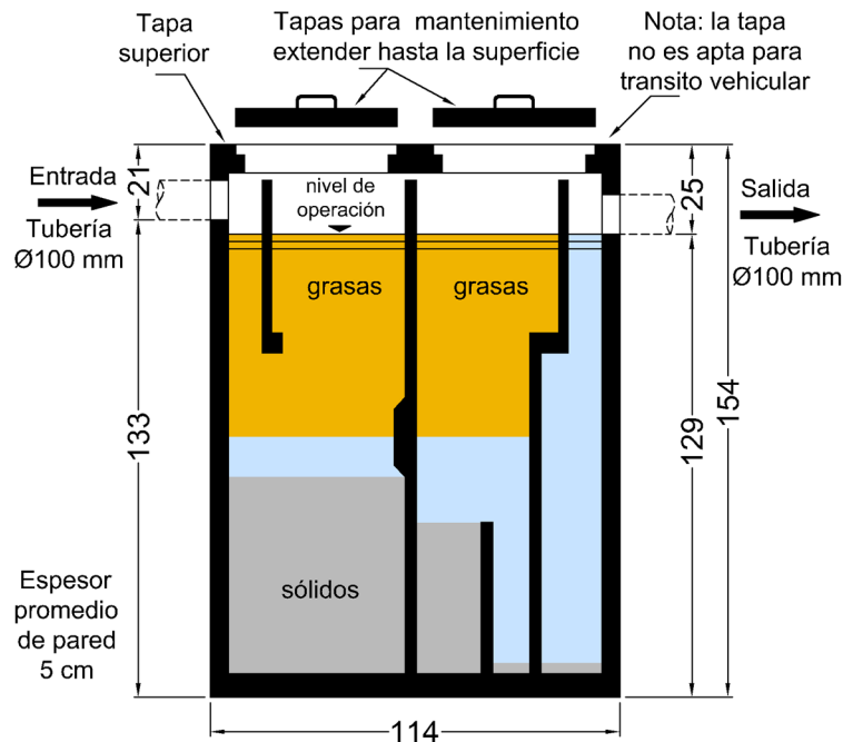
Interceptor de Grasas y Sólidos T.D. Modelo IGS-003 sección vertical - medidas en cm
