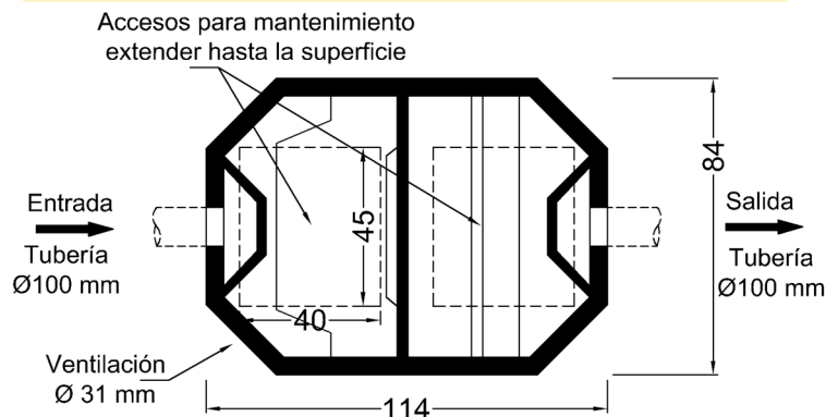
Interceptor de Grasas y Sólidos T.D. Modelo IGS-001 sección horizontal - medidas en cm
