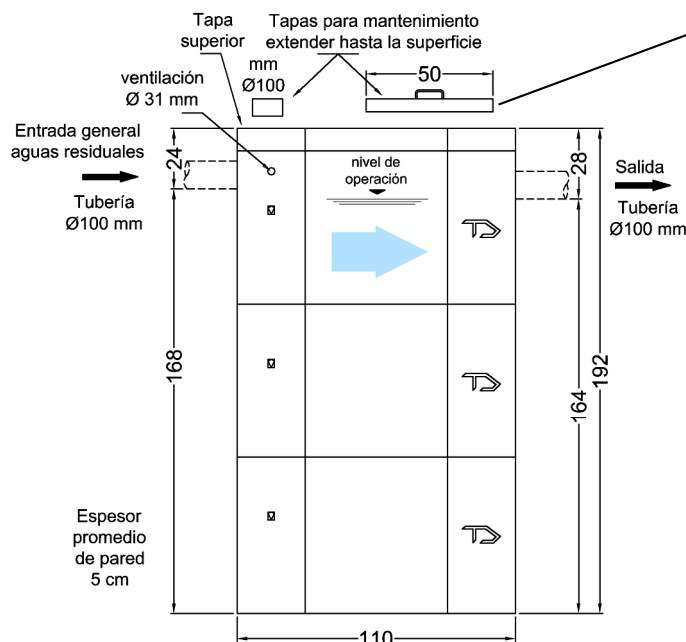
Fosa Biológica T.D. - Modelo FB-30 XL volumen de funcionamiento 1,5 M³ vista vertical - medidas en cm ©TANQUE DIEZ - Derechos Reservados
