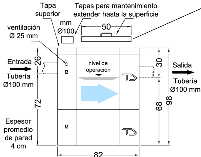
Fosa Biológica T.D. Modelo FB-3 vista vertical - medidas en cm
