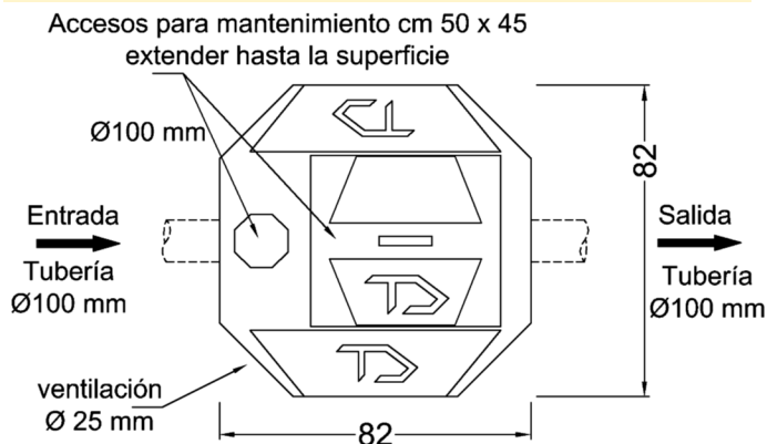
Fosa Biológica T.D. Modelo FB-3 vista superior - medidas en cm
