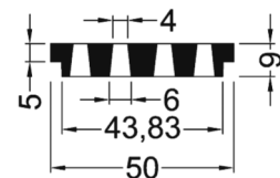
Tapa de rejilla en concreto para Caja Multiuso T.D. sección A-A - medidas en cm
