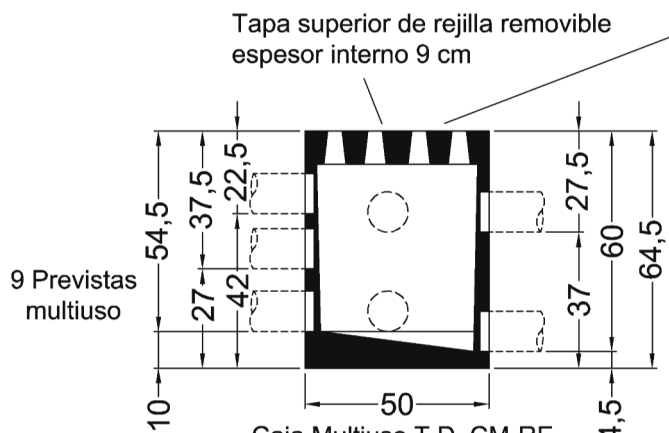
Caja Multiuso T.D. CM-RE tapa de rejilla en concreto sección vertical - medidas en cm
