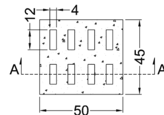
Tapa de rejilla en concreto para Caja Multiuso T.D. vista superior - medidas en cm
