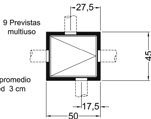
Caja Multiuso T.D. CM-RE tapa de rejilla en concreto sección horizontal - medidas en cm
